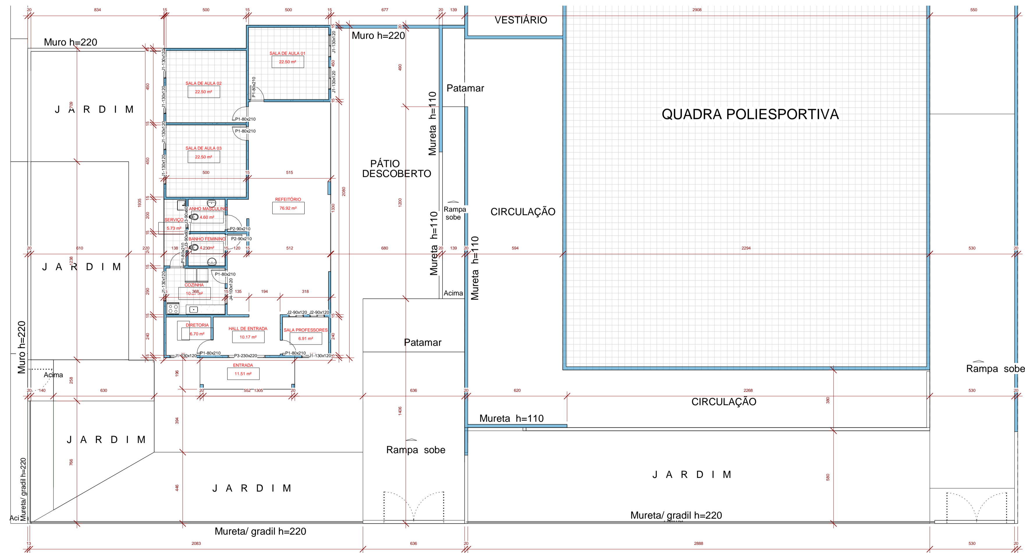
1º PAVIMENTO 1:125
