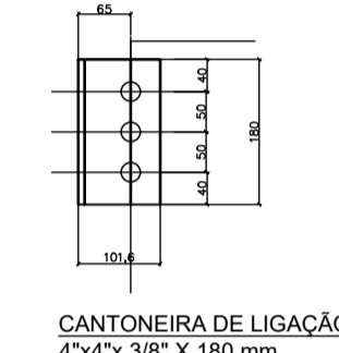
CANTONEIRA DE LIGAÇÃO 4"x4"x 3/8" X 180 mm
