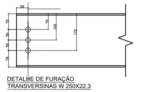
DETALHE DE FURAÇÃO TRANSVERSINAS W 250X22.3
