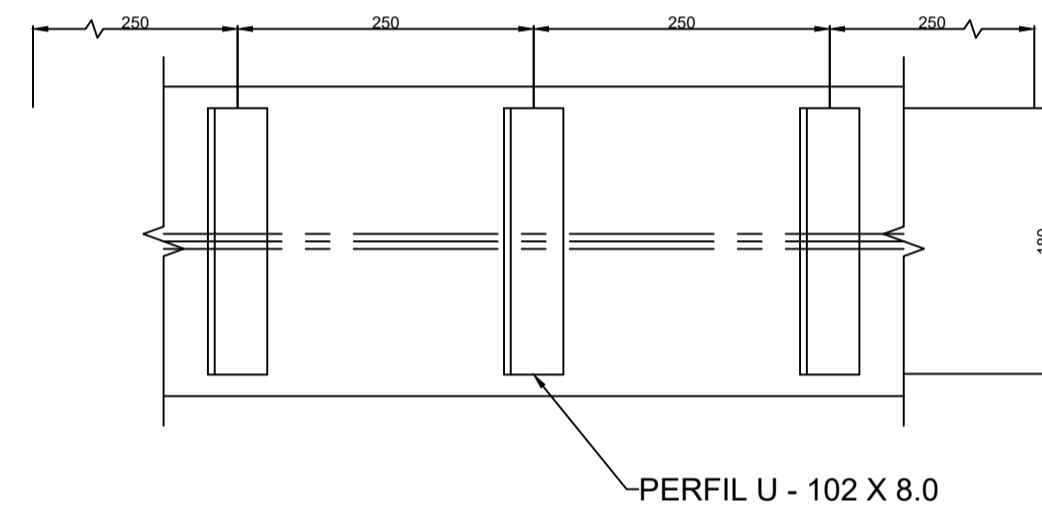
LOCAÇÃO DOS CONECTORES
