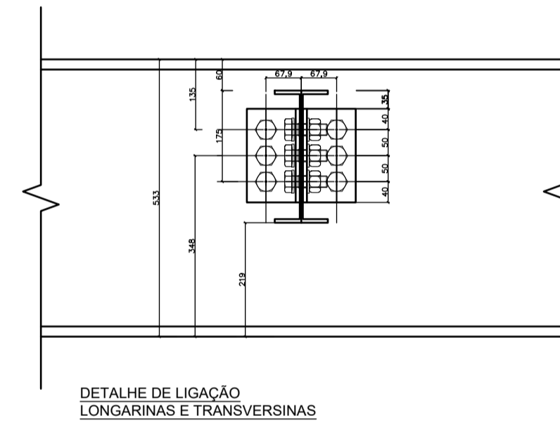
DETALHE DE LIGAÇÃO LONGARINAS E TRANSVERSINAS
