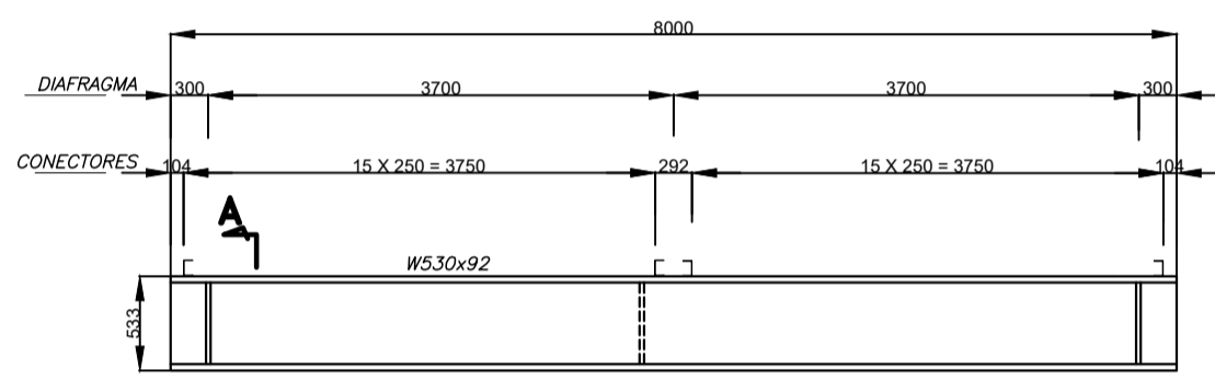
DETALHE DA LONGARINA
