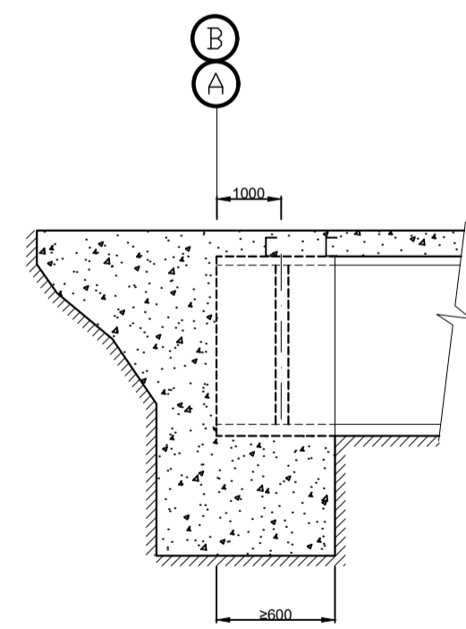
DETALHE DO ENCONTRO
