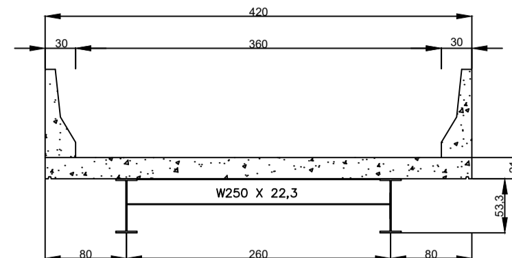
SEÇÃO TRANSVERSAL
