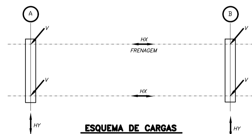
ESQUEMA DE CARGAS
