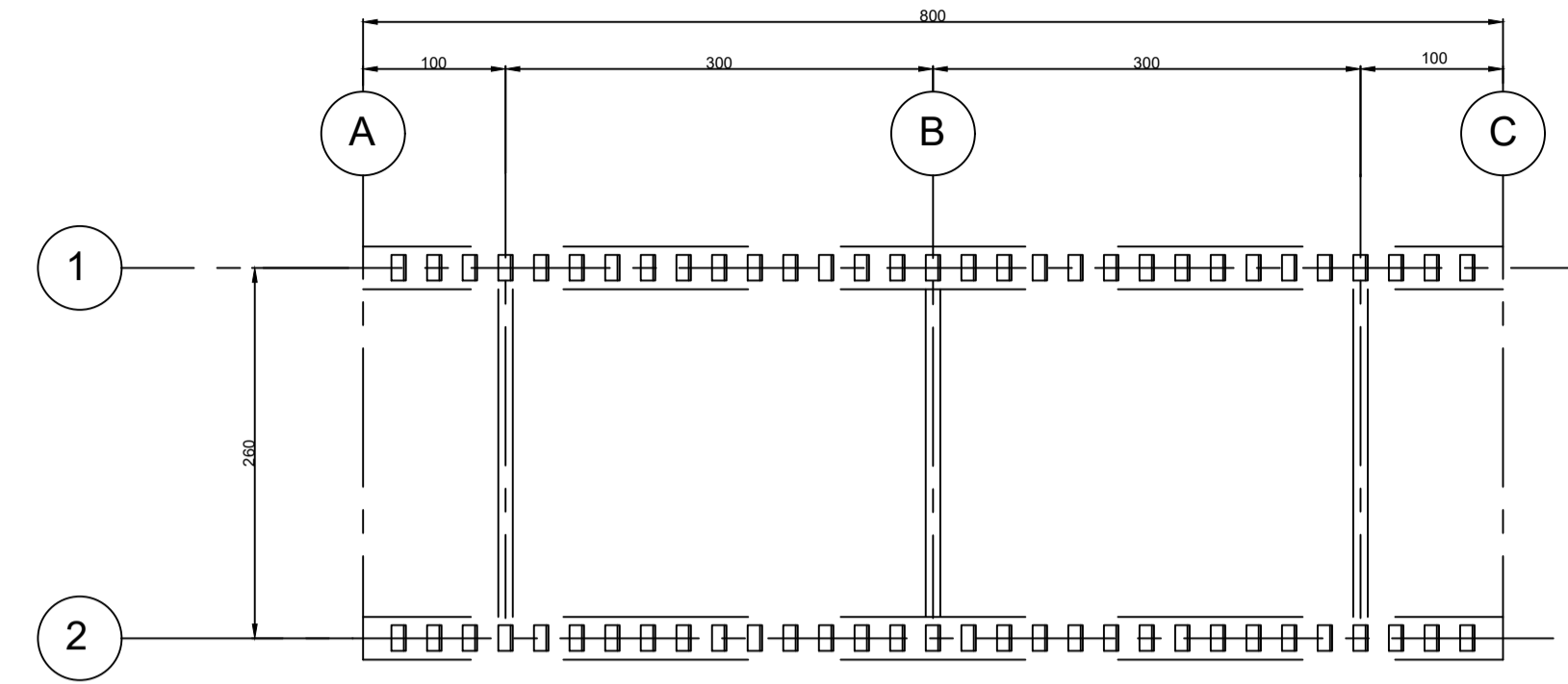
PLANTA BAIXA
