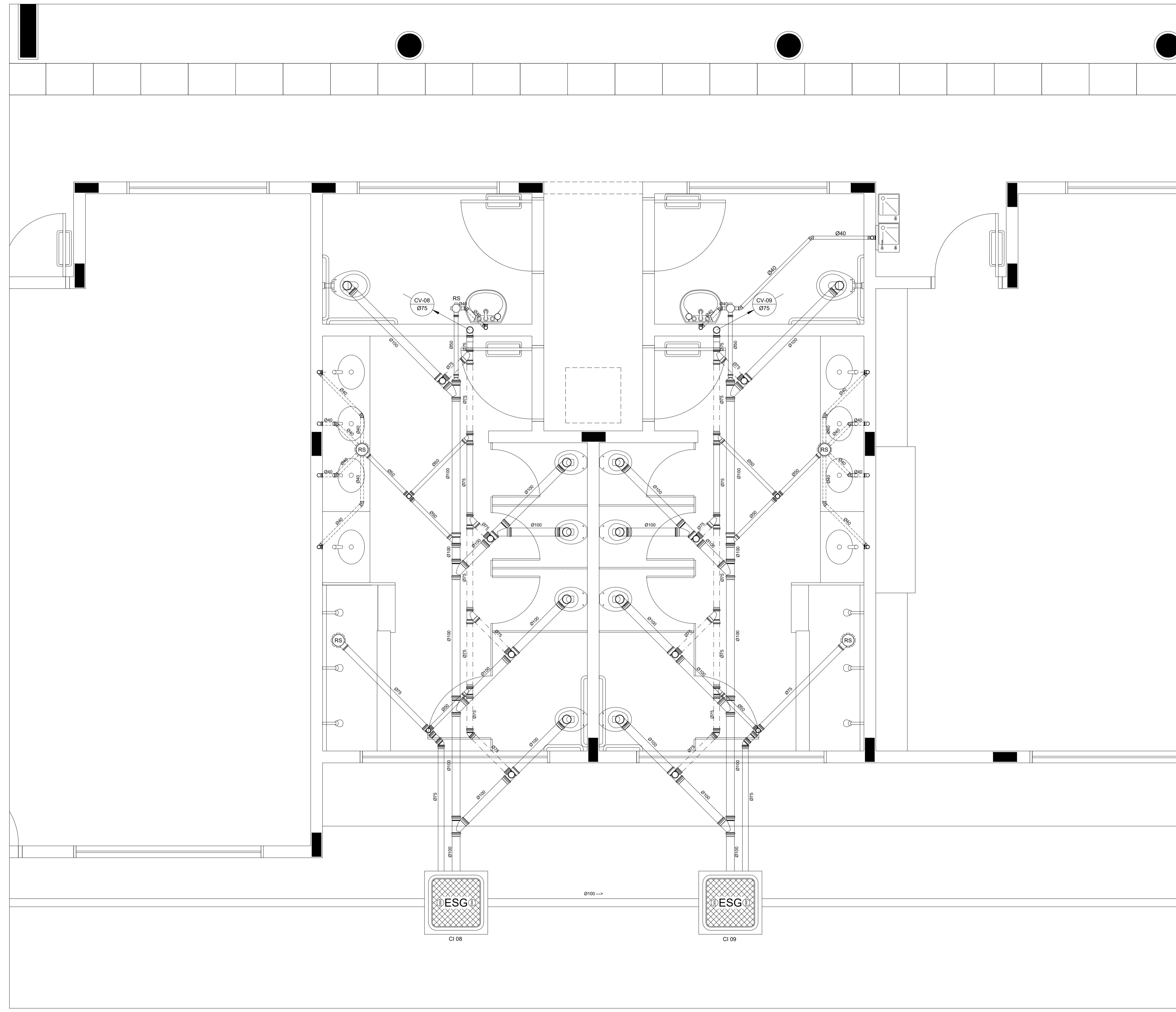
1 AMPLIAÇÃO 05 ESCALA: 1:25
