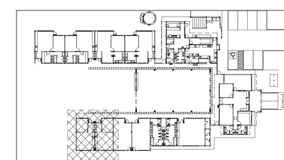
2 PLANTA CHAVE ESCALA: 1/500
