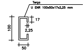
DETALHE DAS TERÇAS
