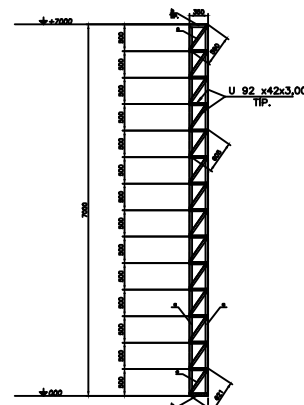
ELEVÇÃO FILAS 1 A 8 1A & 2A (x16)
