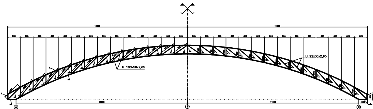
ELEVÇÃO FILAS A/B & C 3A (x8)
