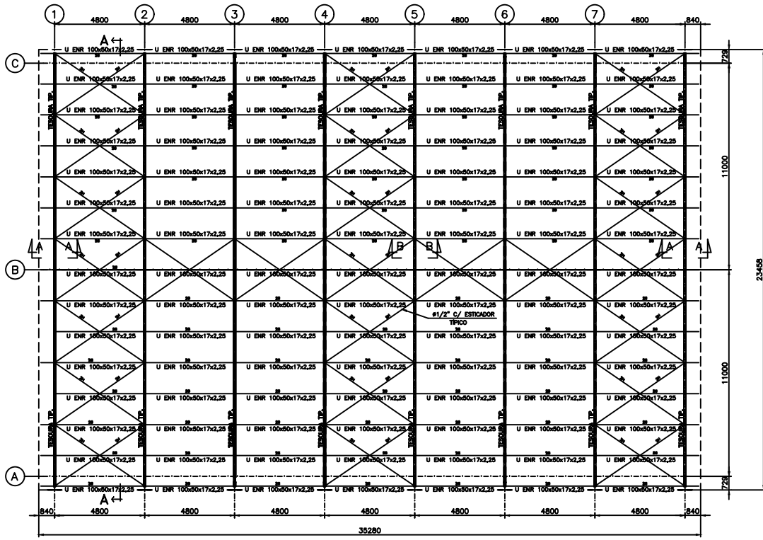
PLANO DA COBERTURA
