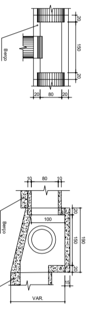
CAIXA DE LIGAÇÃO E PASSAGEM SEM ESCALA
