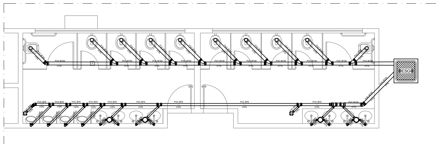
DET. S2 escala 1:25
