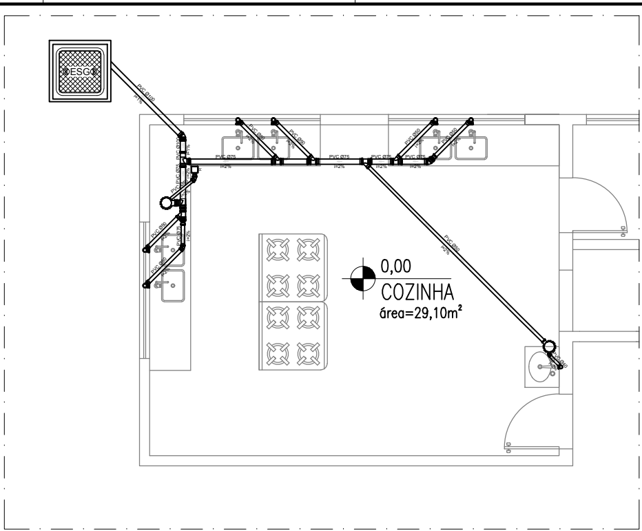
DET. S1 escala 1:25
