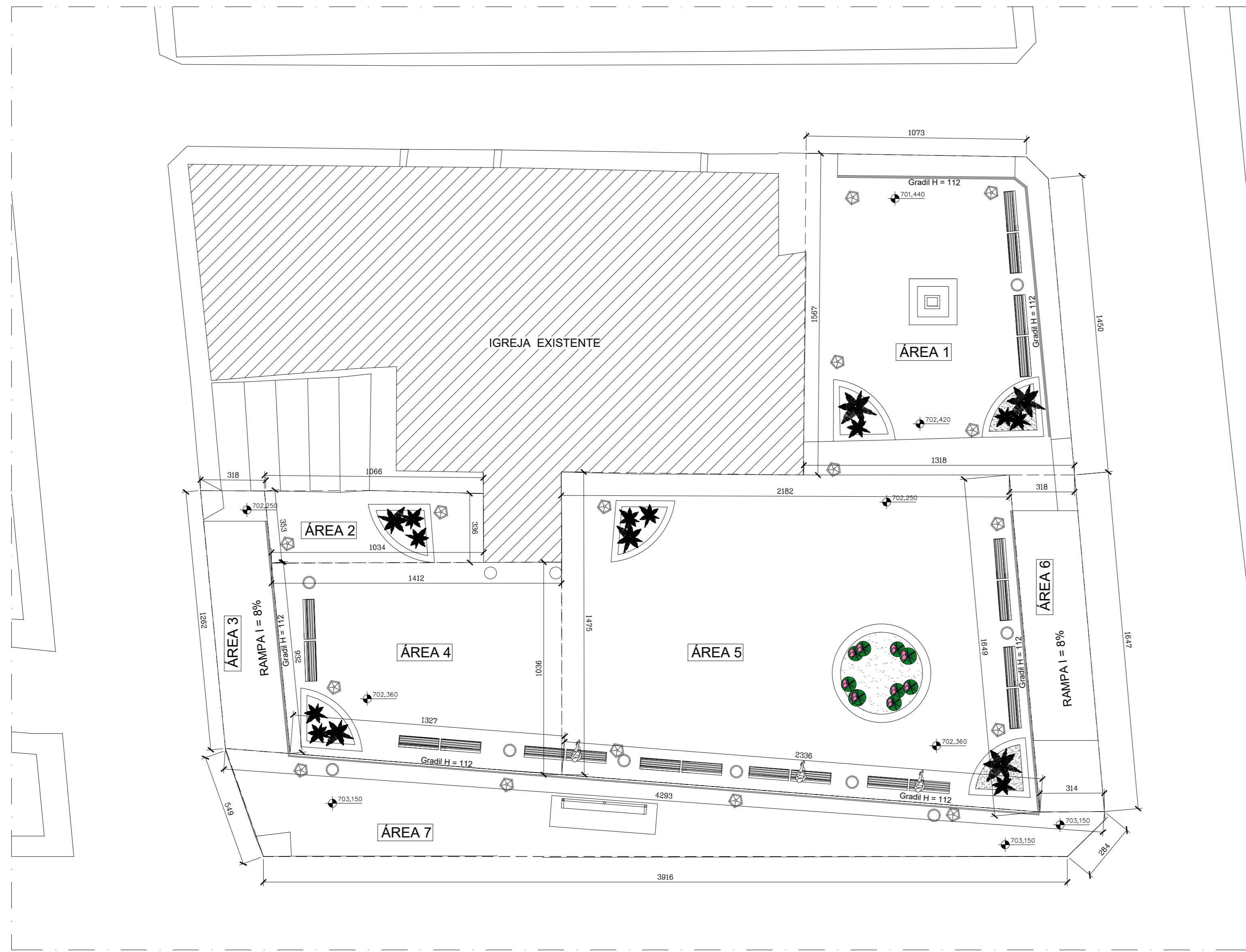
PRAÇA BOM JESUS - PLANTA BAIXA ESCALA: 1/50
