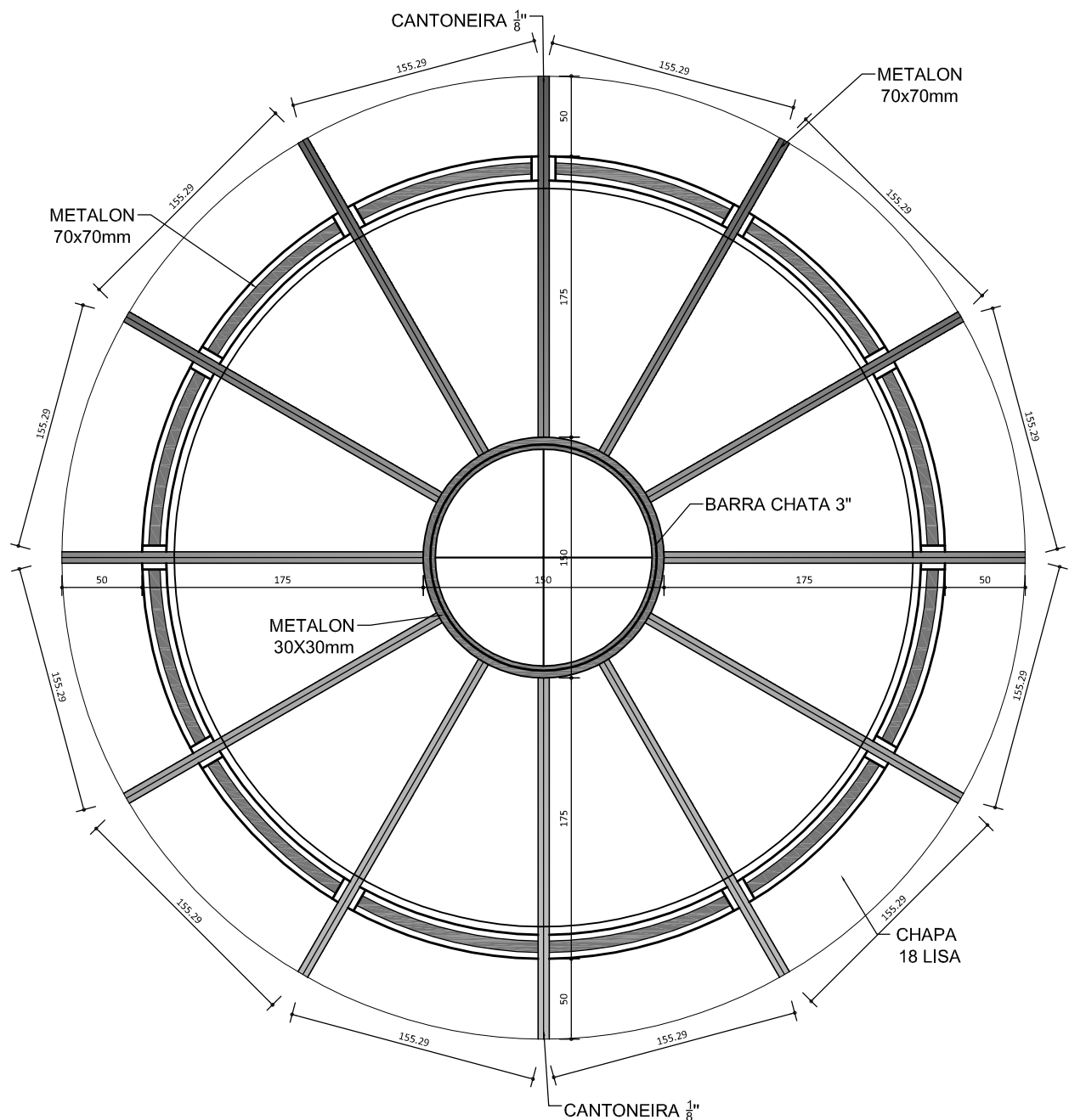
PLANTA CORETO MARILÂNDIA ESCALA 1:40
