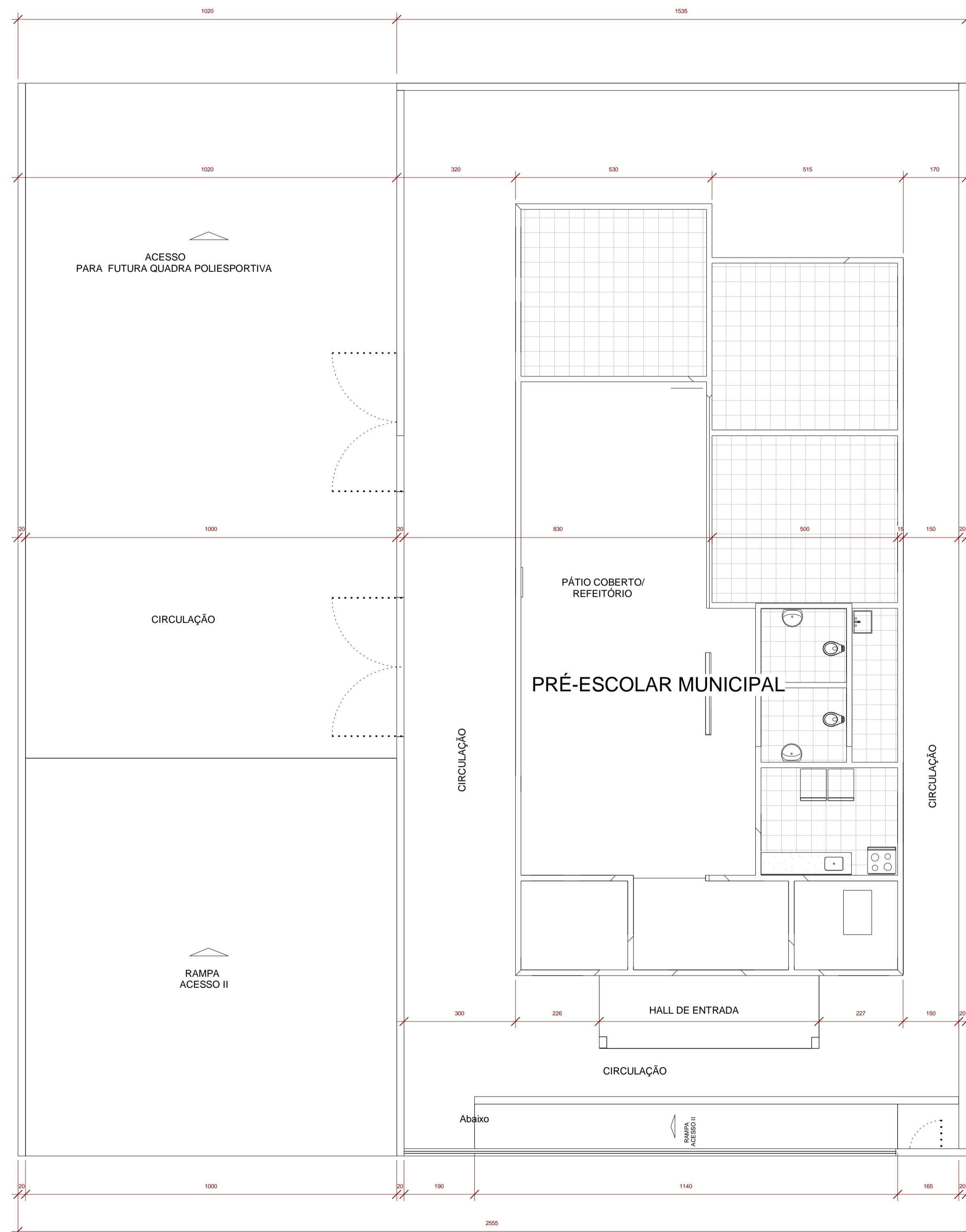
1 PLANTA BAIXA 1 : 75
